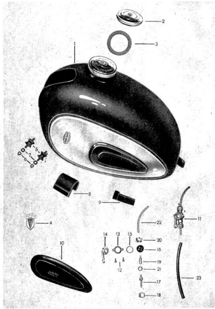
2 — FAHRGESTELL Kraftstoffbehälter, Kraftstoffhahn RT 175 S - RT 200 S / RT 175 VS - RT 200 VS Tafel 27
