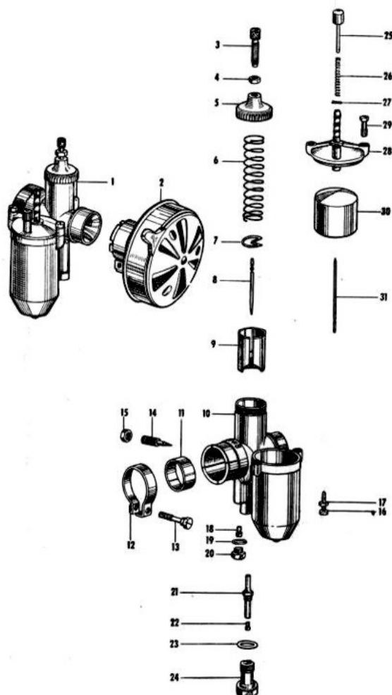
Vergaser RT 125/2 H u. RT 125/2
