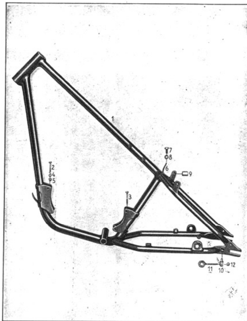
Tafel 12 Gruppe R: a) Rahmen
