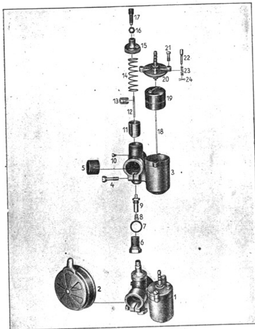
Tafel 7 Gruppe M: d) Vergaser
