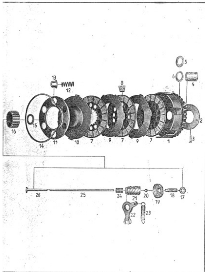
Tafel 8 Gruppe M: e) Kupplung
