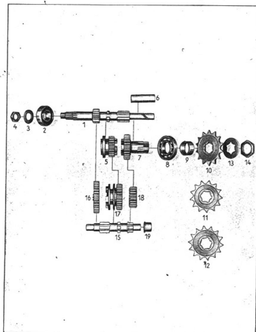
Tafel 9 Gruppe G: a) Wellen- und Zahnräder
