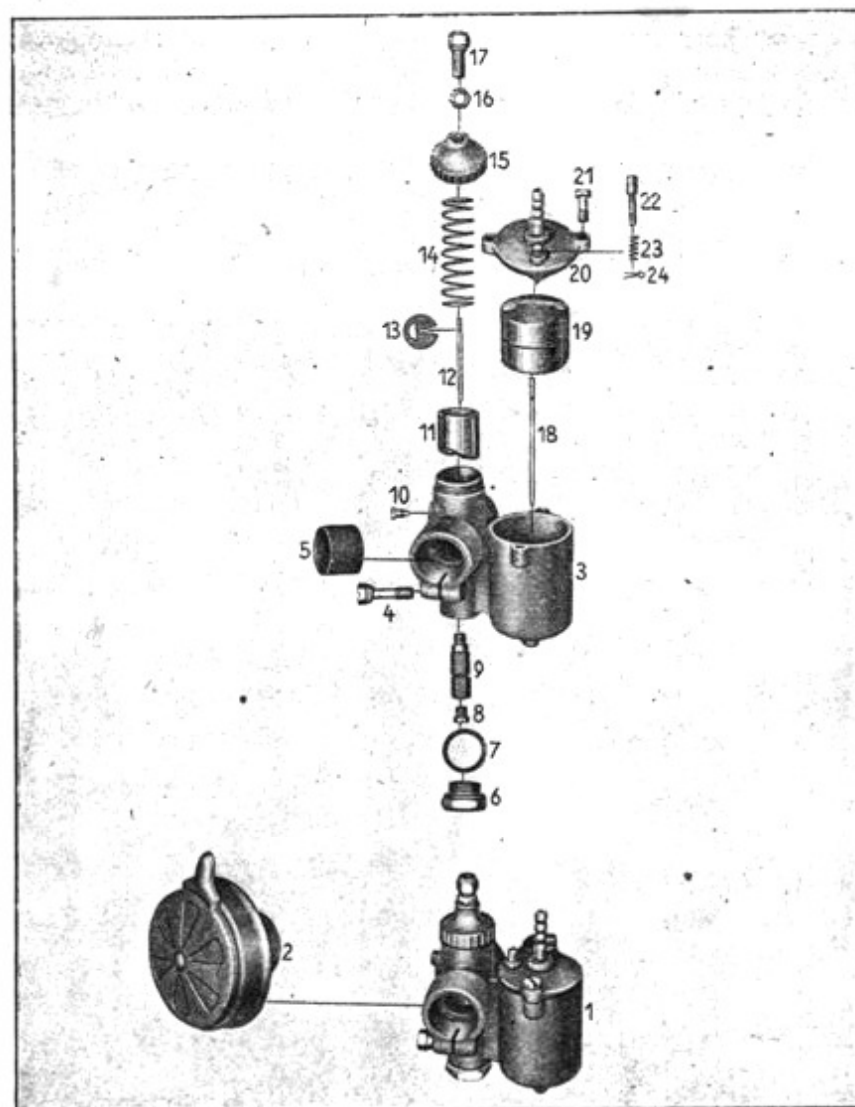
Tafel 5 Gruppe M: d) Vergaser
