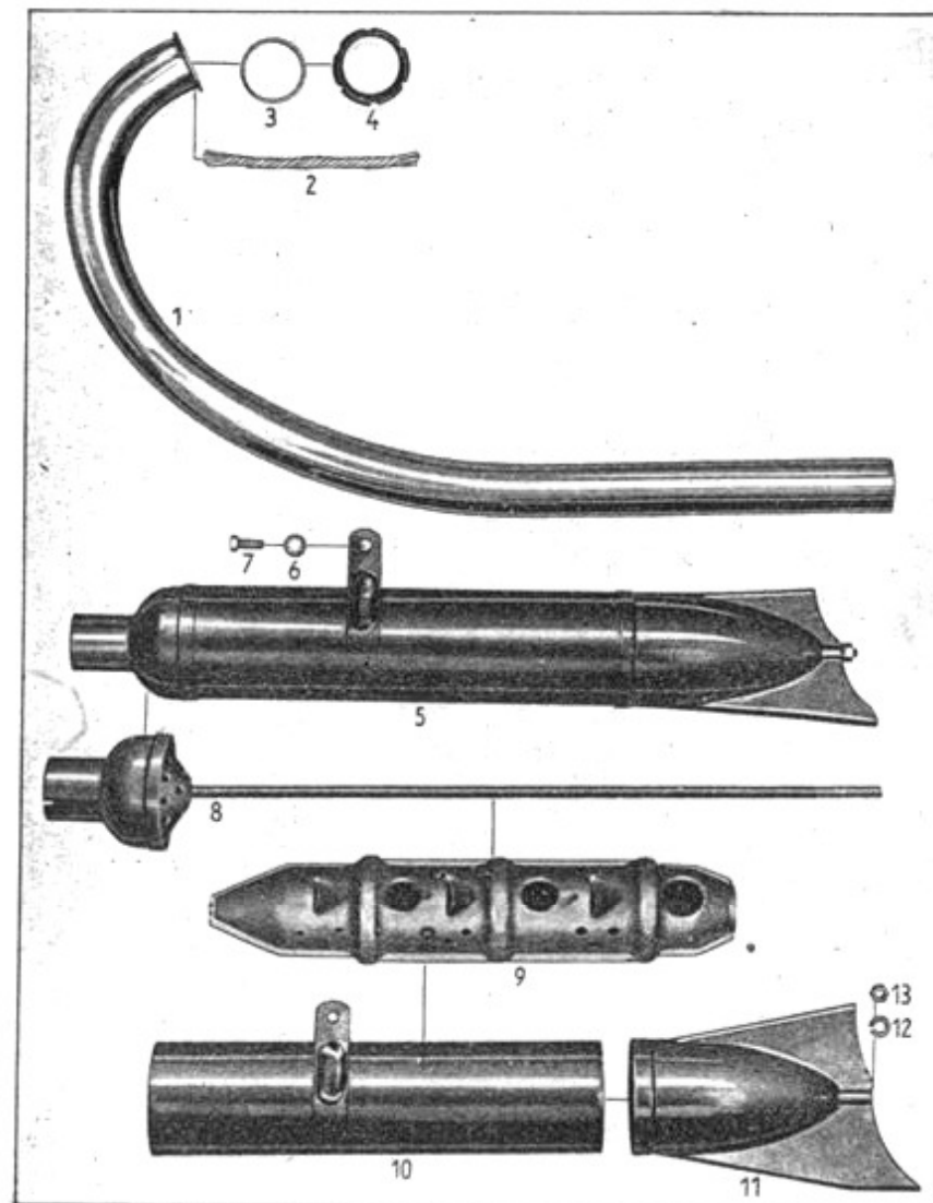
Tafel 17 Gruppe R: h) Auspuffanlage
