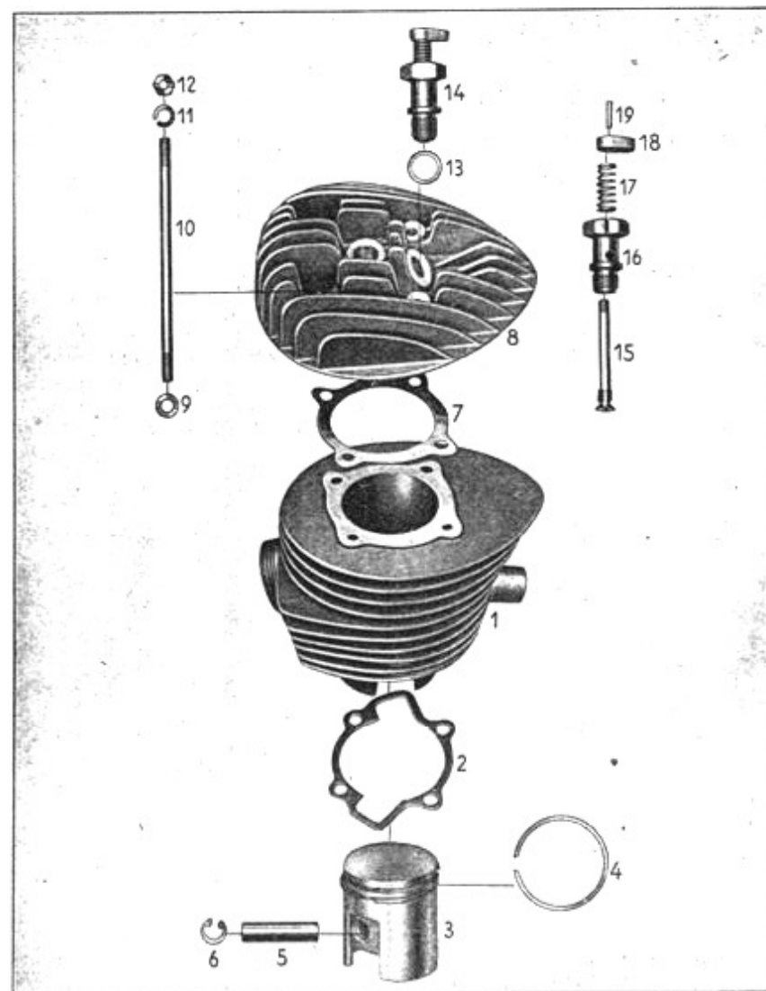
Tafel 3 Gruppe M: b) Zylinder und Kolben
