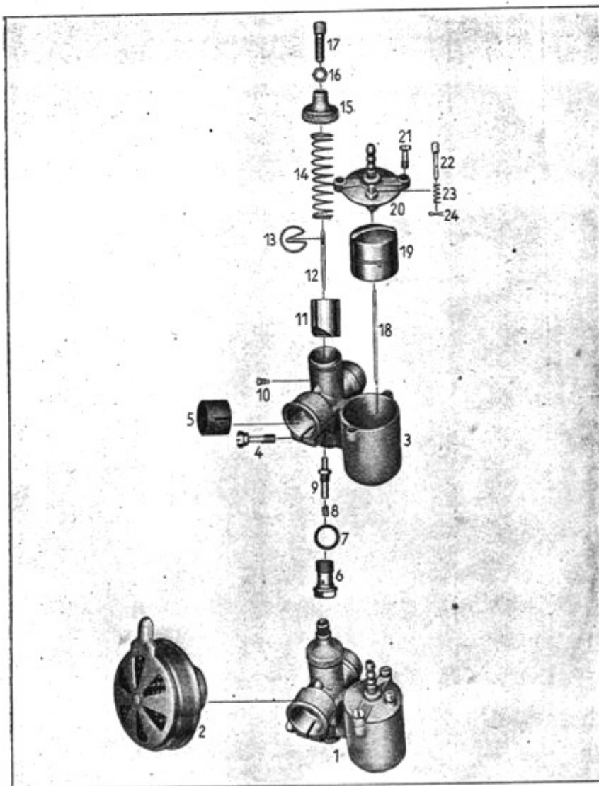
Tafel 6 Gruppe M: d) Vergaser
