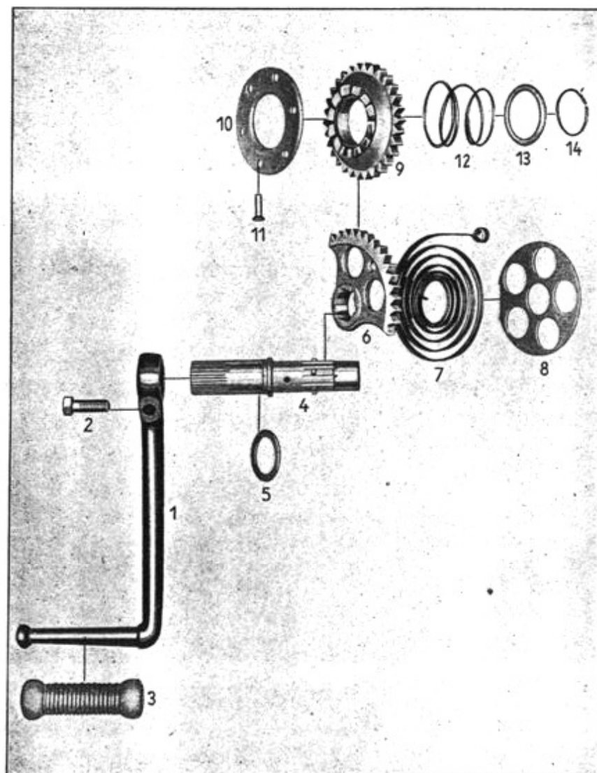
Tafel 11 Gruppe G: c) Kickstarter
