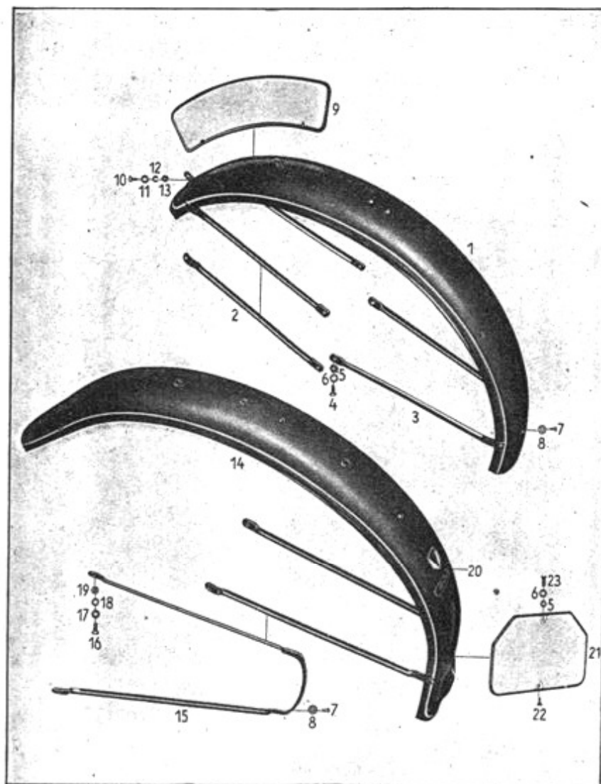
Tafel 15 Gruppe R: d) Kotflügel
