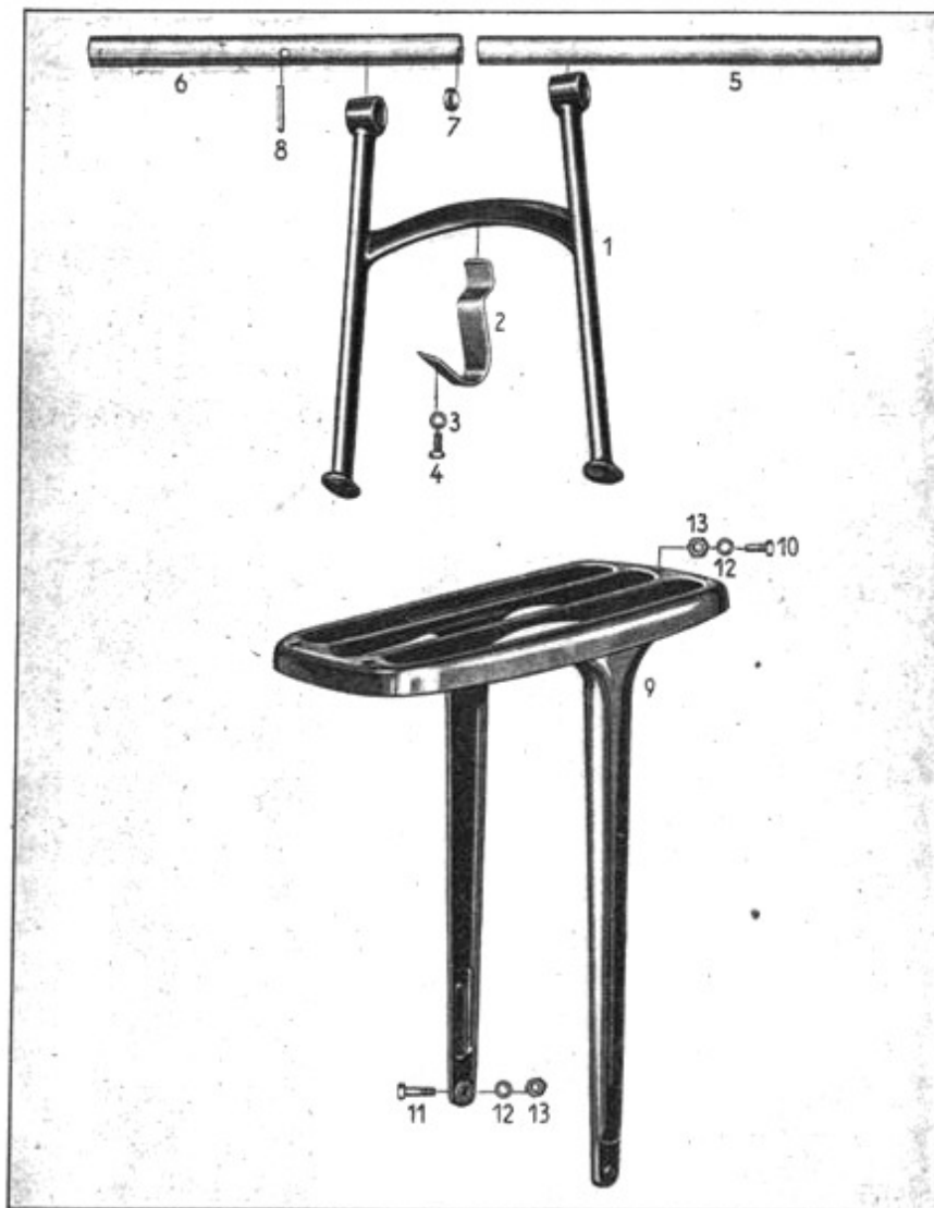
Tafel 14 Gruppe R: c) Gepäckträger und Kippständer
