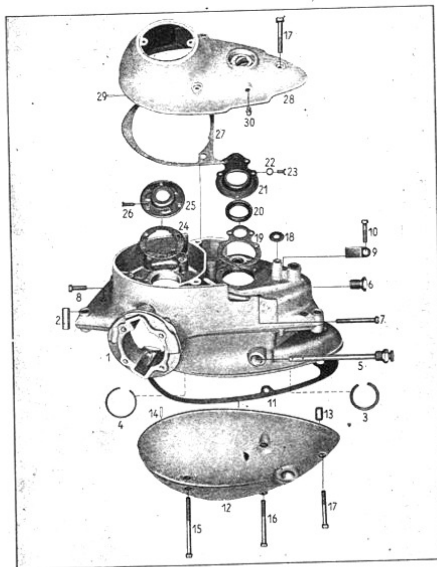
Tafel 2 Gruppe M: a) Motor 2. Motor- und Getriebe Gehäuse
