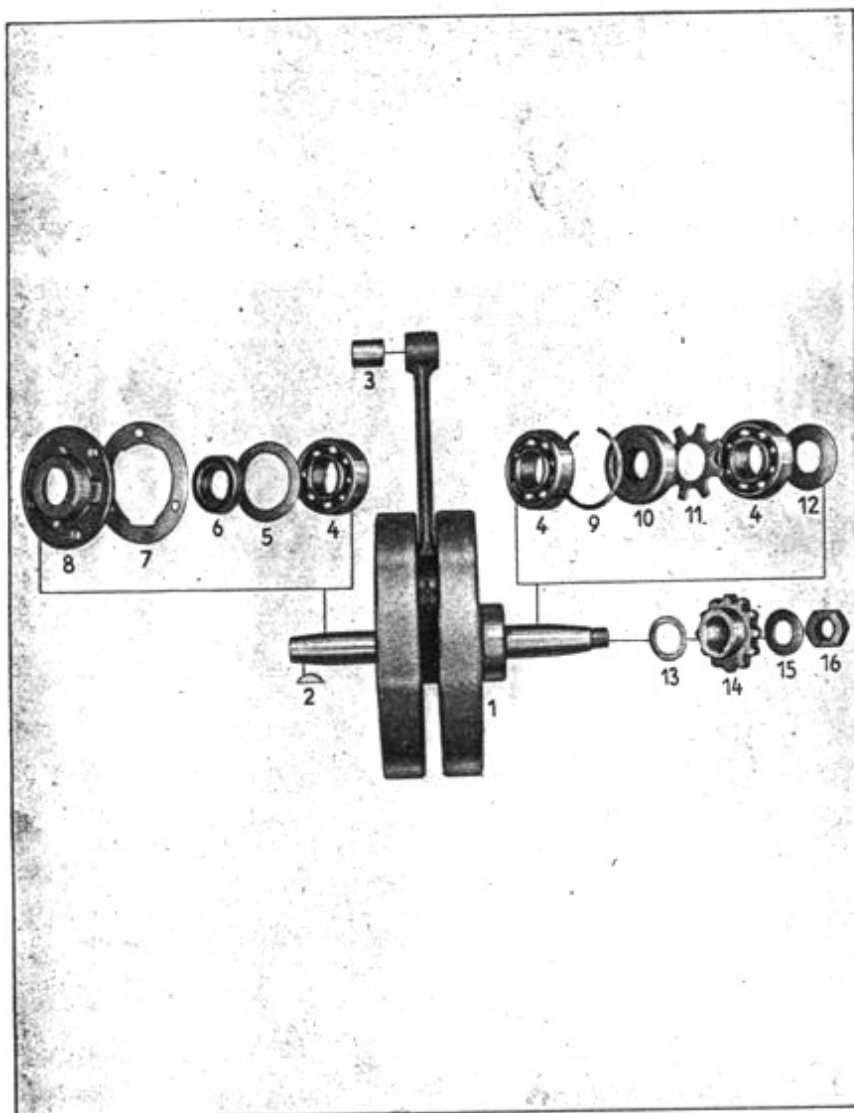
Tafel 4 Gruppe M: c) Triebwerk
