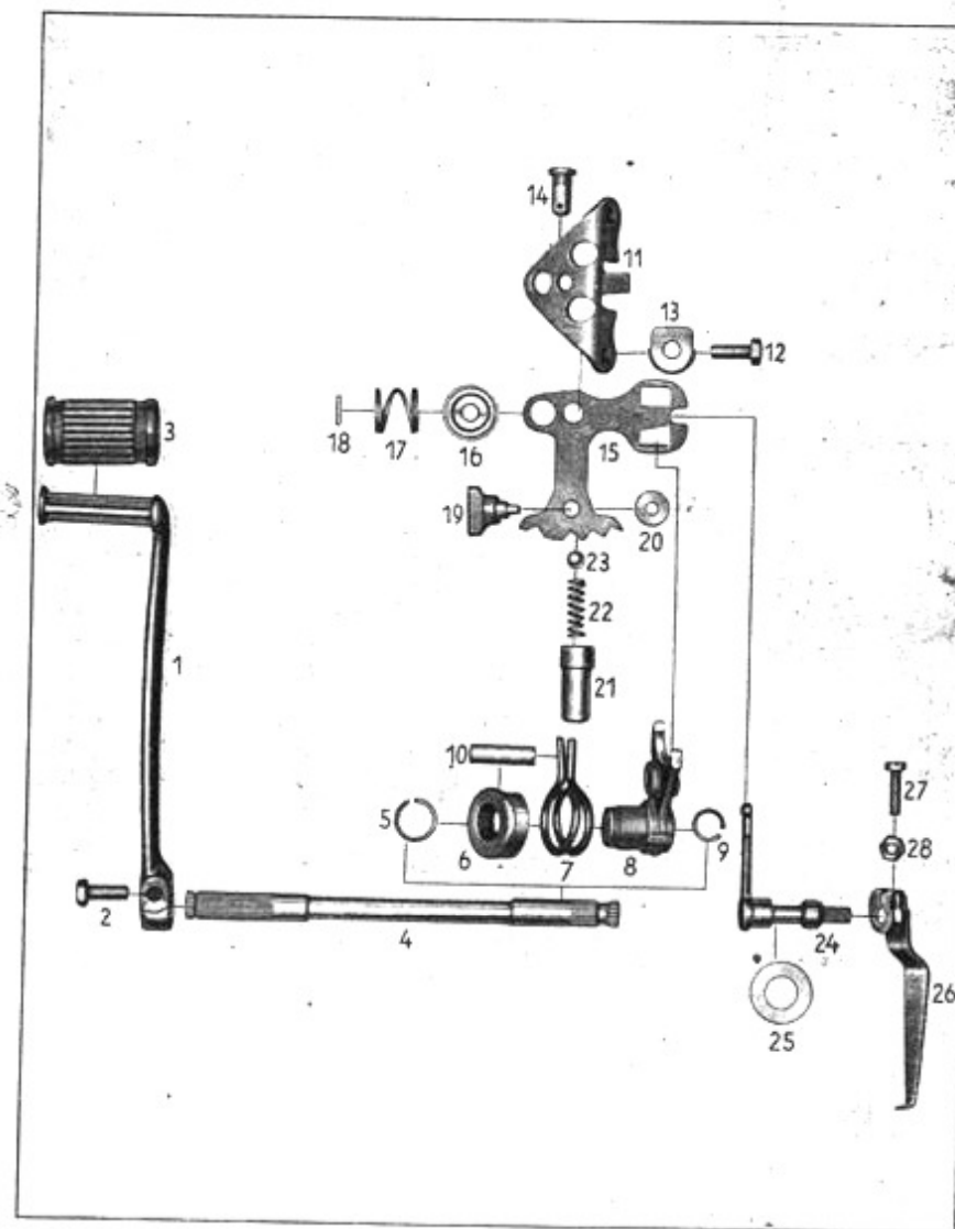
Tafel 10 Gruppe G: b) Gangschaltung
