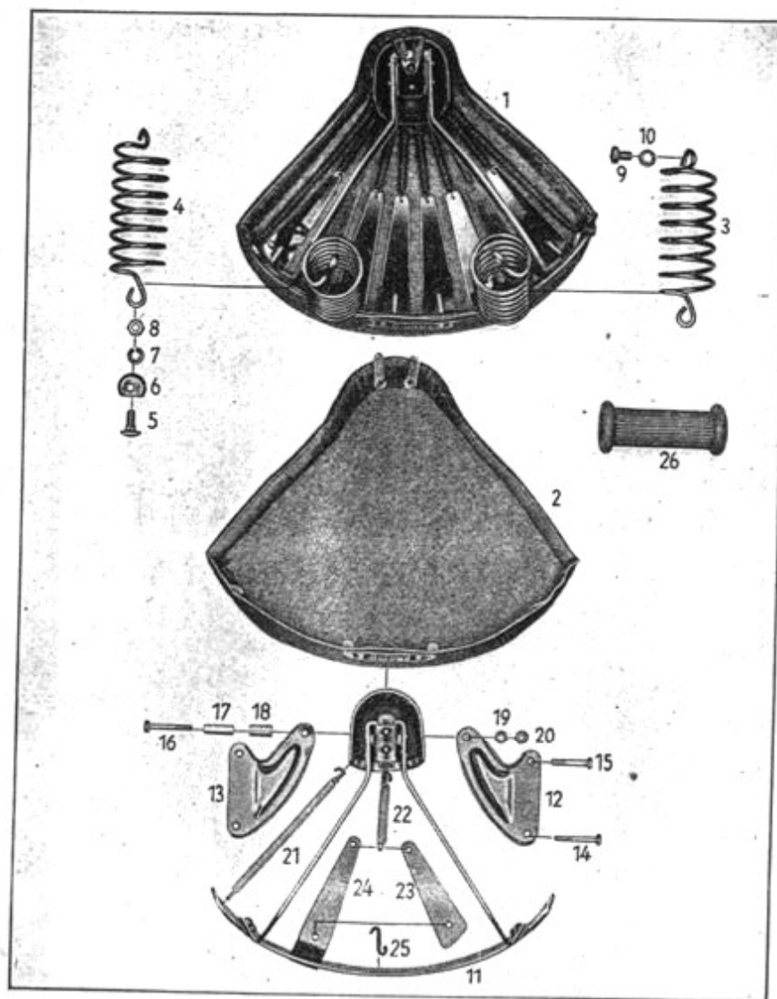
Tafel 13 Gruppe R: b) Sattel, Fußrasten
