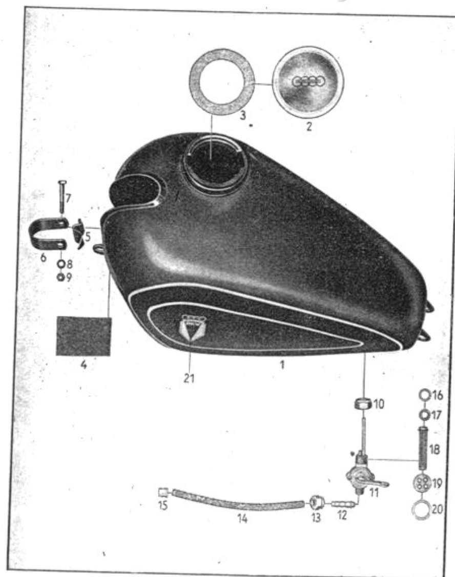
Tafel 16 Gruppe R: f) Kraftstoffbehälter
